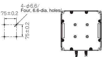
取付穴加工寸法 / Mounting Hole Dimensions
