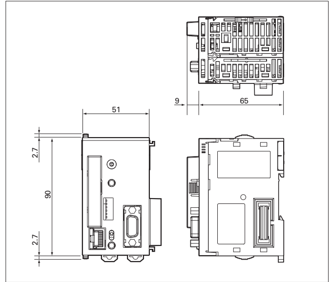
CJ1W-SPU01-V2
